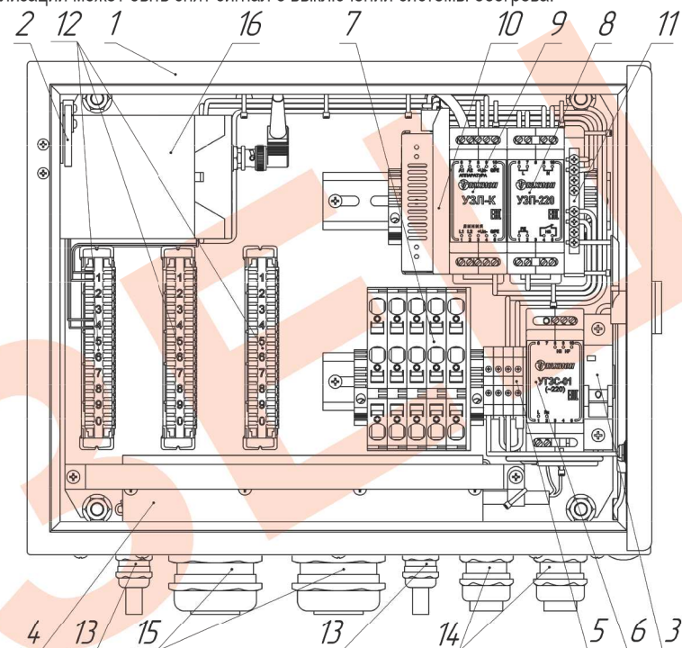
Рис. 1. Устройство термошкафа (дверь открыта на 90°)
